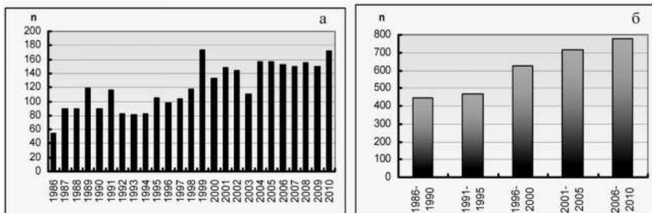
Рисунок 1. Кількість випадків (n) стихійних метеорологічних явищ в окремі роки (а) і п'ятиріччя(б) на території України
